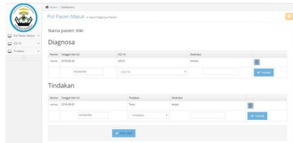
Gambar 12. Halaman Periksa
